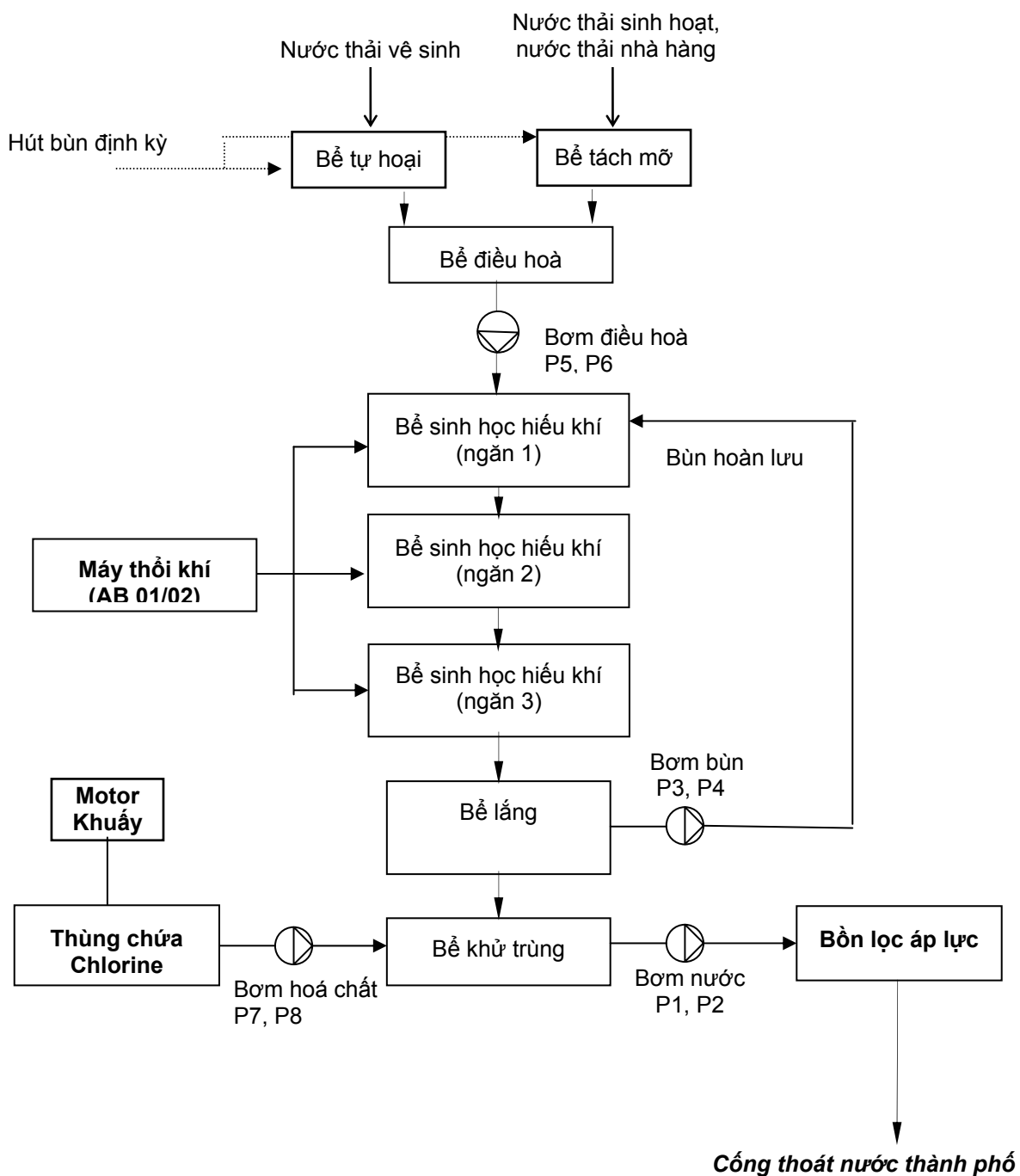
Sơ đồ khối công nghệ xử lý nước thải tập trung khu Tây
