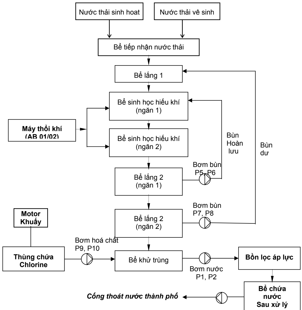
Sơ đồ khối công nghệ xử lý nước thải tập trung khu Mới và khu Đông
